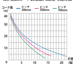
〈表〉延長コード長と最大連結可能灯数
