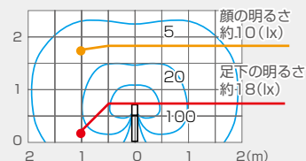
ポールライトの鉛直面照度分布図
