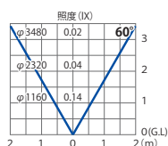
水平面照度分布図
