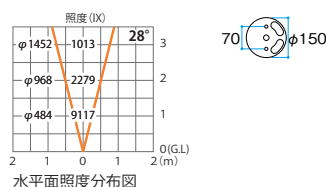
水平面照度分布図
