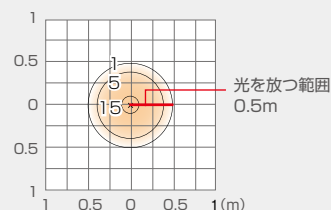
ガーデンバスライト2型の床面照度分布図
