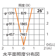
水平面照度分布図
