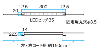
30cm 連結用 寸法図
