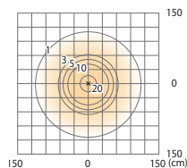
床面照度分布図
