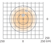
床面照度分布図
