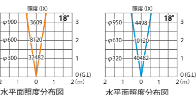
水平面照度分布図
