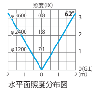
水平面照度分布図
