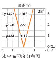
水平面照度分布図
