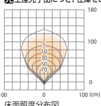
床面照度分布図
