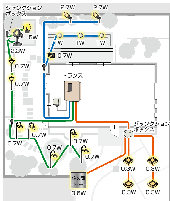
配線レイアウト図
