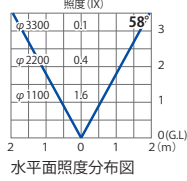
水平面照度分布図
