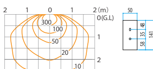
鉛直面照度分布図
