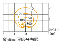
鉛直面照度分布図
