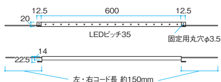
60cm 連結用 寸法図
