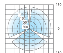
床面照度分布図
