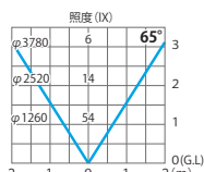
水平面照度分布図
