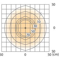
床面照度分布図
