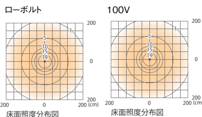
床面照度分布図
