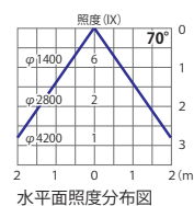
水平面照度分布図
