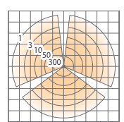
床面照度分布図
