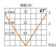
水平面照度分布図
