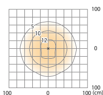
床面照度分布図
